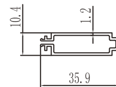
ZYRMQ20010 0.284 kg/m
