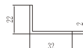
ZYRMQ20016 0.284 kg/m
