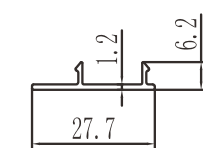
ZYRMQ20006 0.117 kg/m
